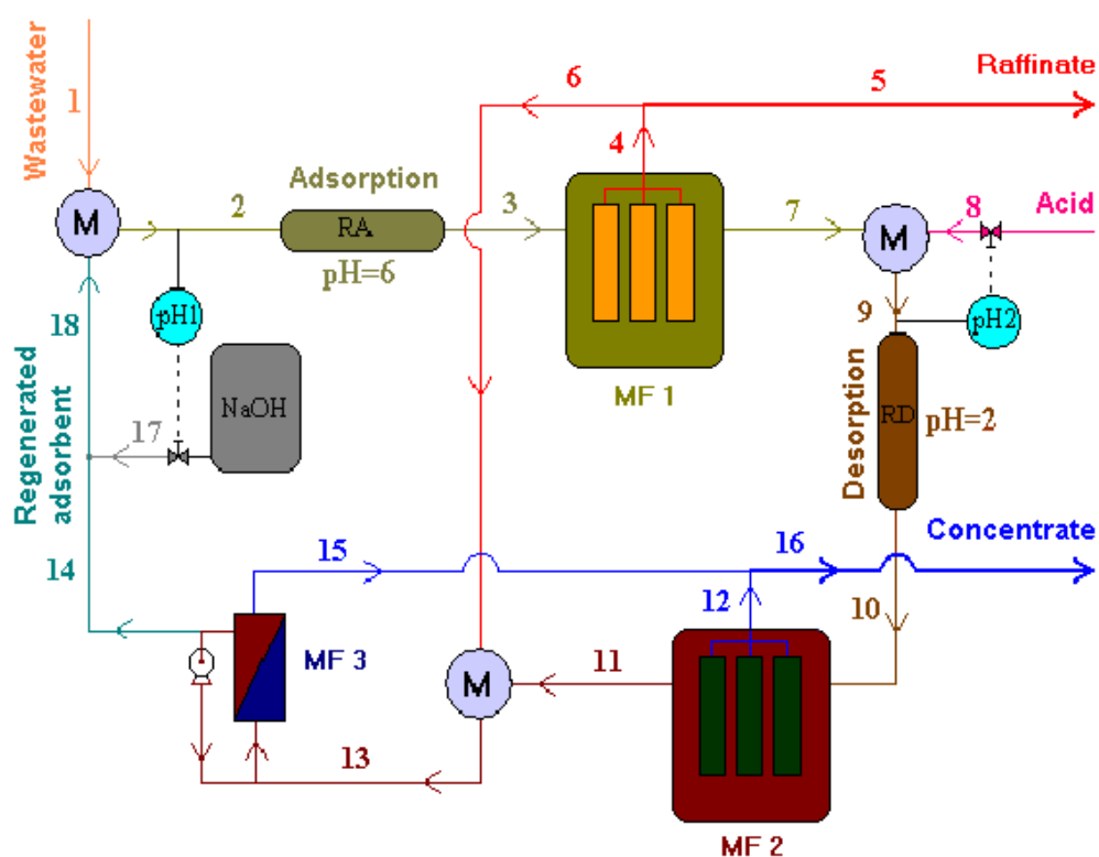
Obr. 11 Schéma hybridného procesu odstraňovania kovov z odpadovej vody
