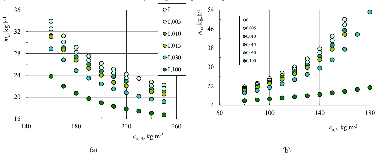
Obr. 12 Vplyv koncentrácie regenerovanej suspenzie (a) a zahustenej suspenzie po adsorpcii (b) na hmotnosť adsorbenta
