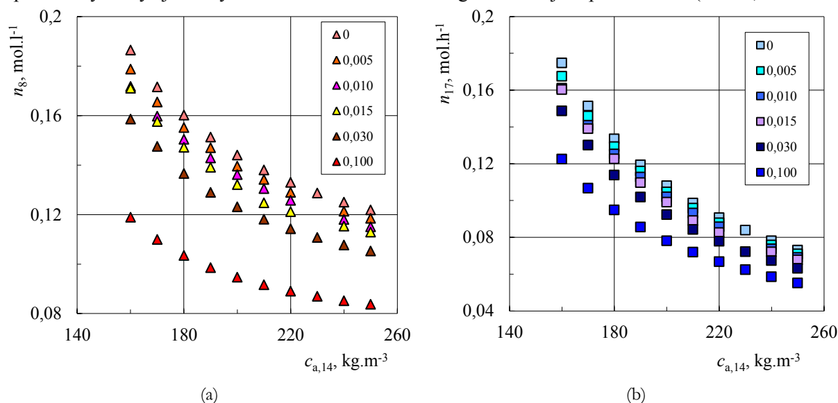
Obr. 4 Vplyv koncentrácie regenerovanej suspenzie na spotrebu a) kyseliny, b) zásady
