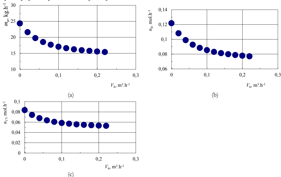
Obr. 5 Vplyv toku spätného premývania na a) hmotnosť adsorbenta, b) spotrebu kyseliny a c) spotrebu zásady
