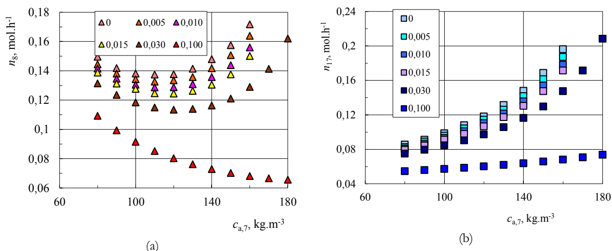
Obr. 13 Vplyv koncentrácie zahustenej suspenzie po adsorpcii na spotrebu a) kyseliny, b) zásady
